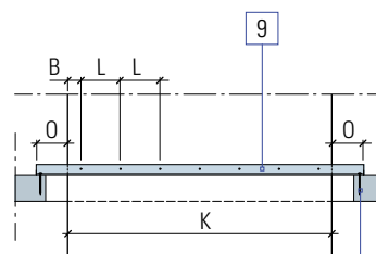
O EI 30 = 120 mm / EI 60 = 175 mm K Dimensions du conduit B Distance du bord L Distance
