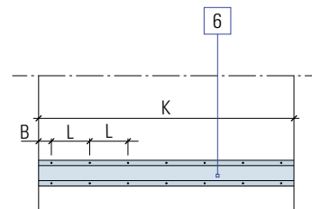
K Dimensions du conduit B Distance du bord L Distance
